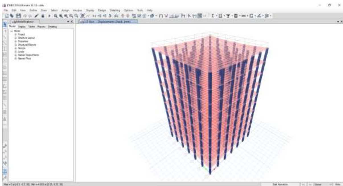
Fig 15 Dead Load
